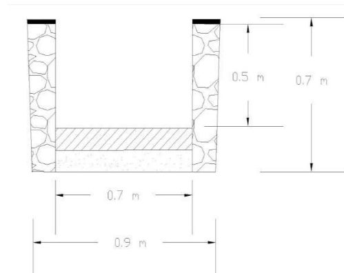
Gambar 16. Drainase Rencana Jalan Bawal
