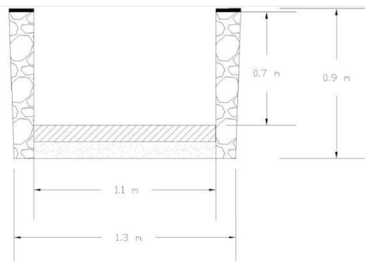
Gambar 11. Drainase Eksisting Jalan Rambutan Depan Jalan Nanas
