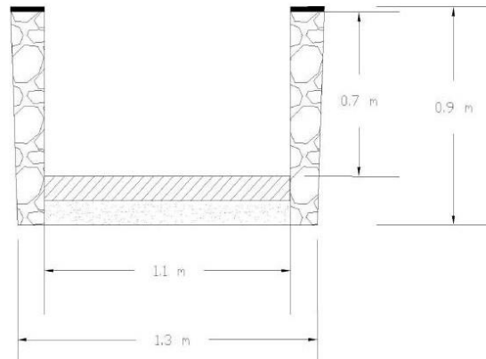
Gambar 12. Drainase Rencana Jalan Rambutan Depan Jalan Nanas
