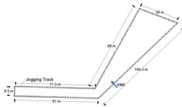
Gambar 10. Skema tampak atas kolam retensi 1 skenario 2
